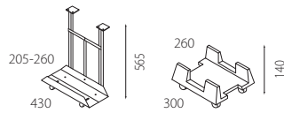
LA 92 AA 31 półka lub podstawa pod komputer CPU-Halter oder CPU-Wagen suspended or mobile CPU-holder
